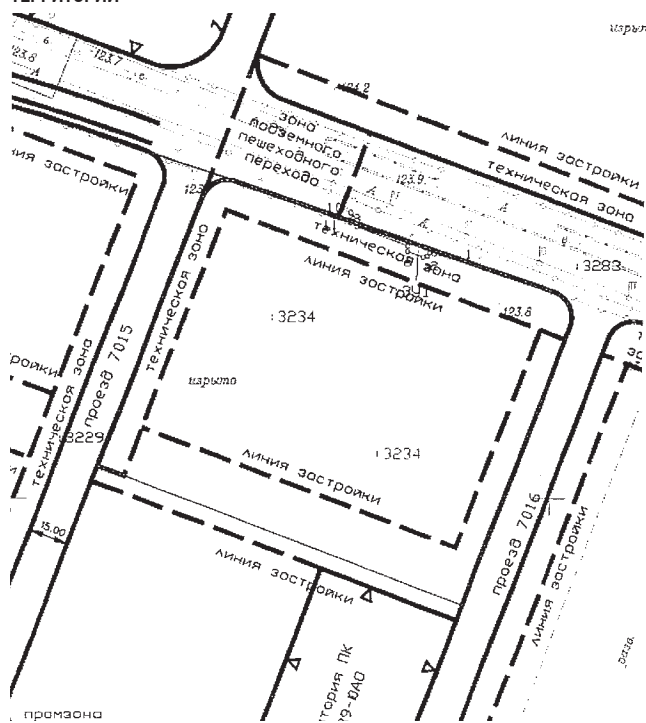
СХЕМА РАСПОЛОЖЕНИЯ ЗЕМЕЛЬНОГО УЧАСТКА НА КАДАСТРОВЫХ ПЛАНАХ ТЕРРИТОРИИ
