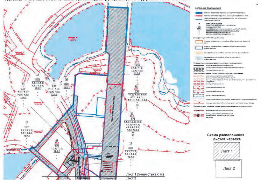
План "Функционально-планировочная организация территории" и План "Границы зон планируемого размещения объектов" Чертеж 2 "Линейные объекты инженерной инфраструктуры и улично-дорожной сети", М 1:2000
