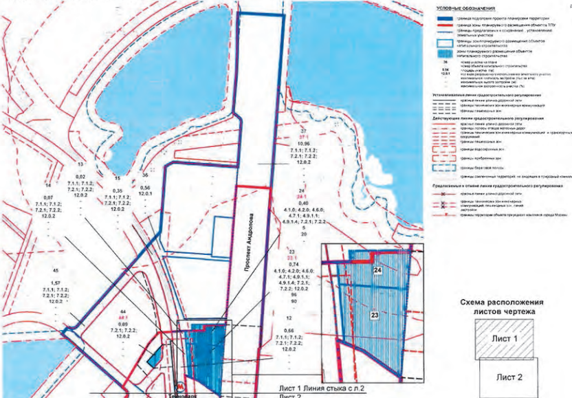
План "Функционально-планировочная организация территории" и План "Границы зон планируемого размещения объектов" Чертеж 1 "Объекты капитального строительства", М 1:2000
