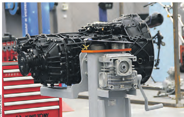
Механическая коробка передач в лаборатории Технологического колледжа
